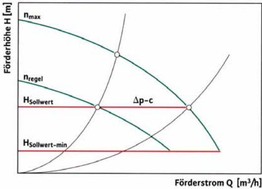
\Delta p - c - Differenzdruck konstant
