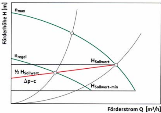
\Delta p - v - Differenzdruck variabel
